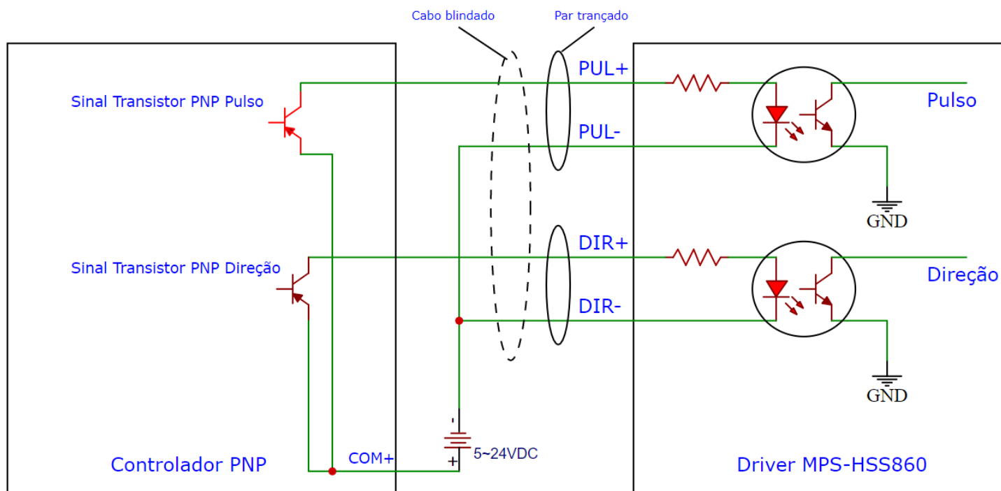
Imagem 3 - Ligação PNP do driver
