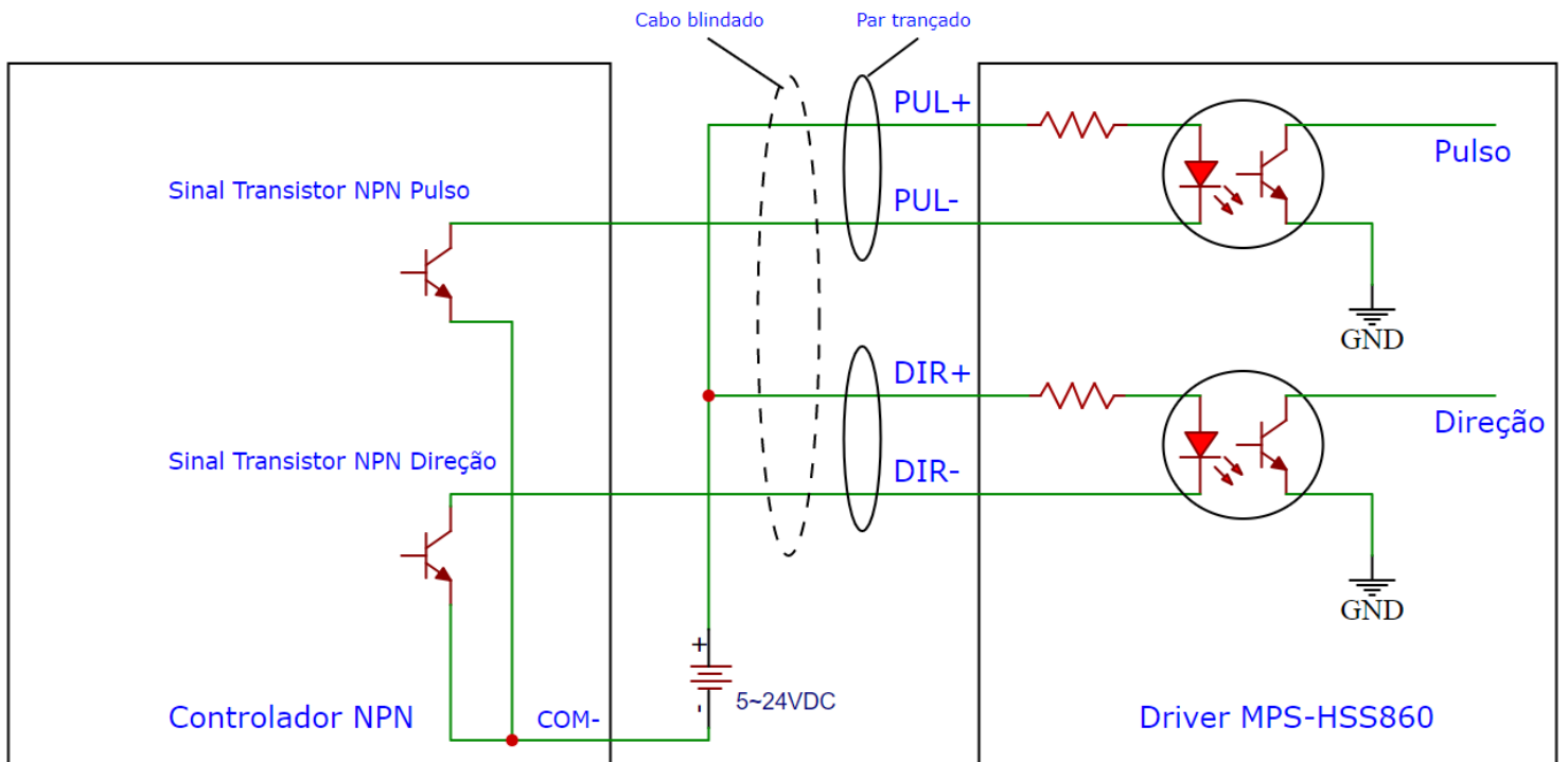
Imagem 2 - Ligação NPN do driver
