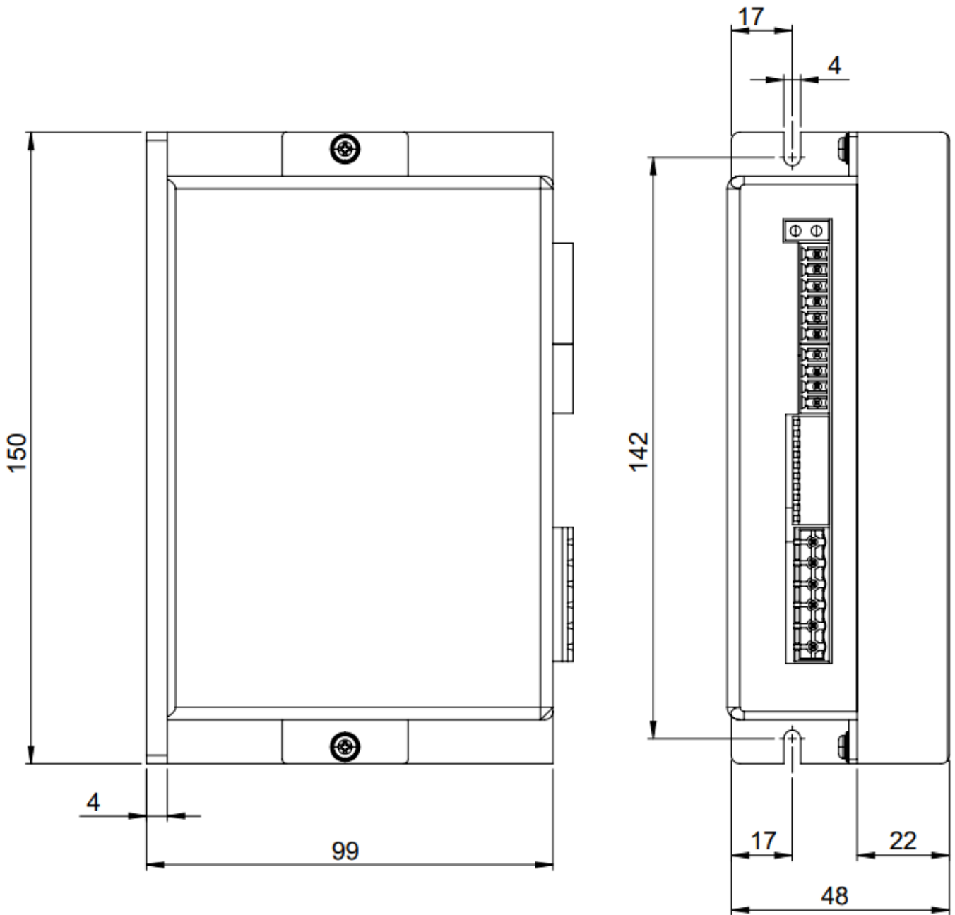
Imagem 1 - Desenhos técnicos do driver
